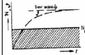
Şekil 12.19. Sürekli işletme N, Nominal güç, u sıcaklık değişimi, t zaman
